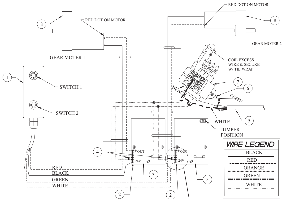
WIRING SCHEMATIC C
